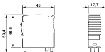
Maßzeichnung
