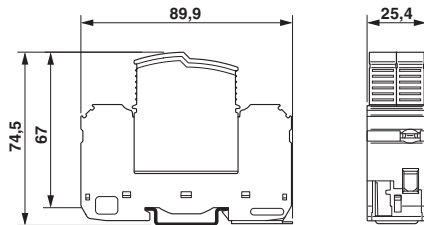
Maßzeichnung
