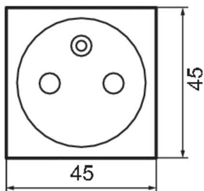
Maßzeichnung
