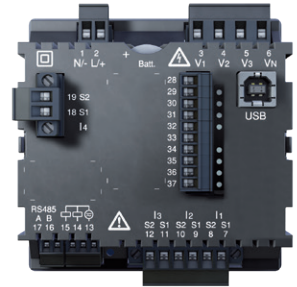
UMG 96RM-CBM
