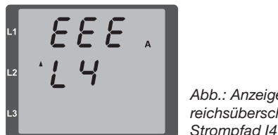
Abb.: Anzeige Messbereichsüberschreitung im Spannungspfad L3.
