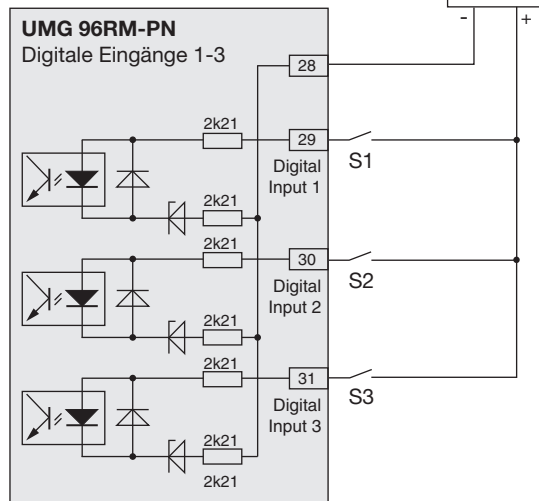
Abb. Beispiel für den Anschluss der externen Schaltkontakte S1 und S2 an die digitalen Eingänge 1 und 2.
