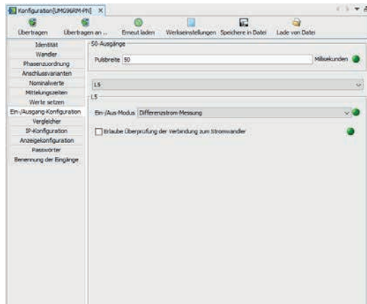
Abb.: Software GridVis, Konfigurationsmenü
