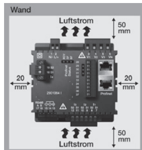
Abb. Einbaulage UMG 96RM-PN (Ansicht von hinten)
