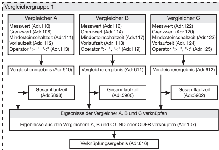
Abb.: Vergleichers-Prinzip der Vergleicherguppe 1
