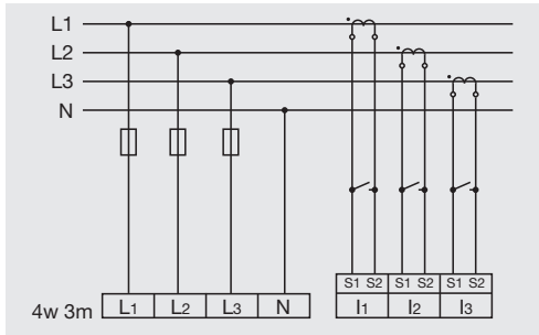
Abb. Messung in einem Dreiphasen-4-Leiternetz mit unsymmetrischer Belastung.
