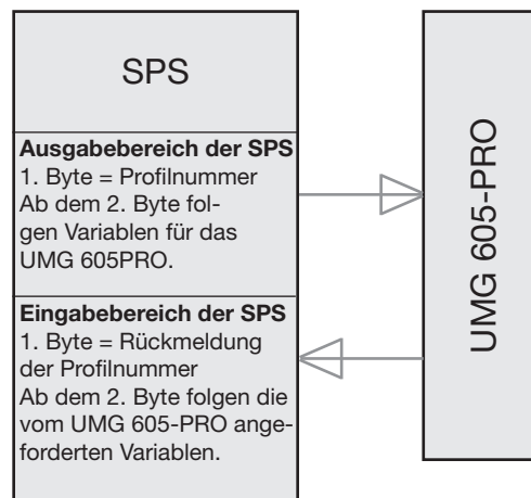
Abb. Blockschaltbild für den Datenaustausch zwischen SPS und UMG 605-PRO.
