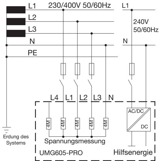
Abb. Prinzipschaltbild, UMG 605-PRO im TN-Netz
