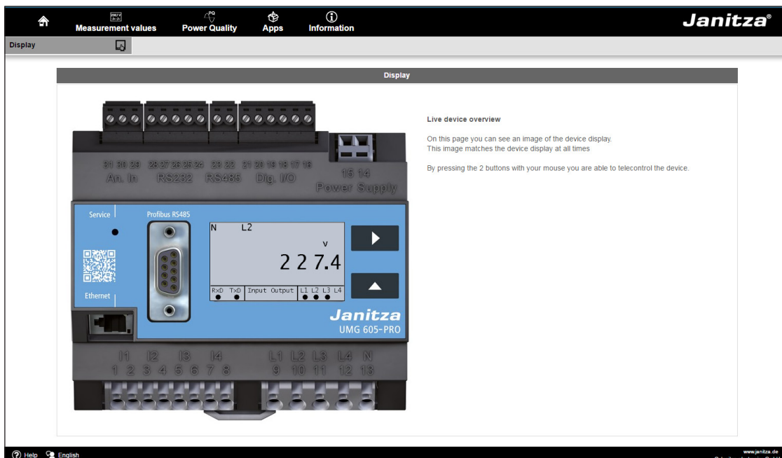
Abb. Bedienung des UMG 605-PRO über die Gerätehomepage
