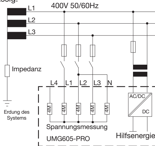
Abb. Prinzipschaltbild, UMG 605-PRO im IT-Netz ohne N.
