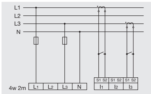
Abb. Messung in einem Dreiphasen-4-Leiternetz mit symmetrischer Belastung.
