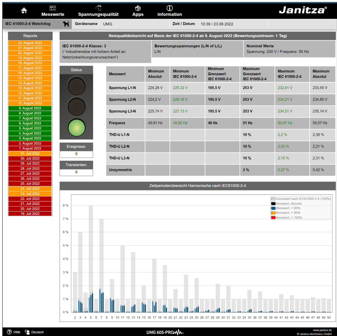
Abb. IEC 61000-2-4 Watchdog Parameter mit Ampelprinzip - Report
