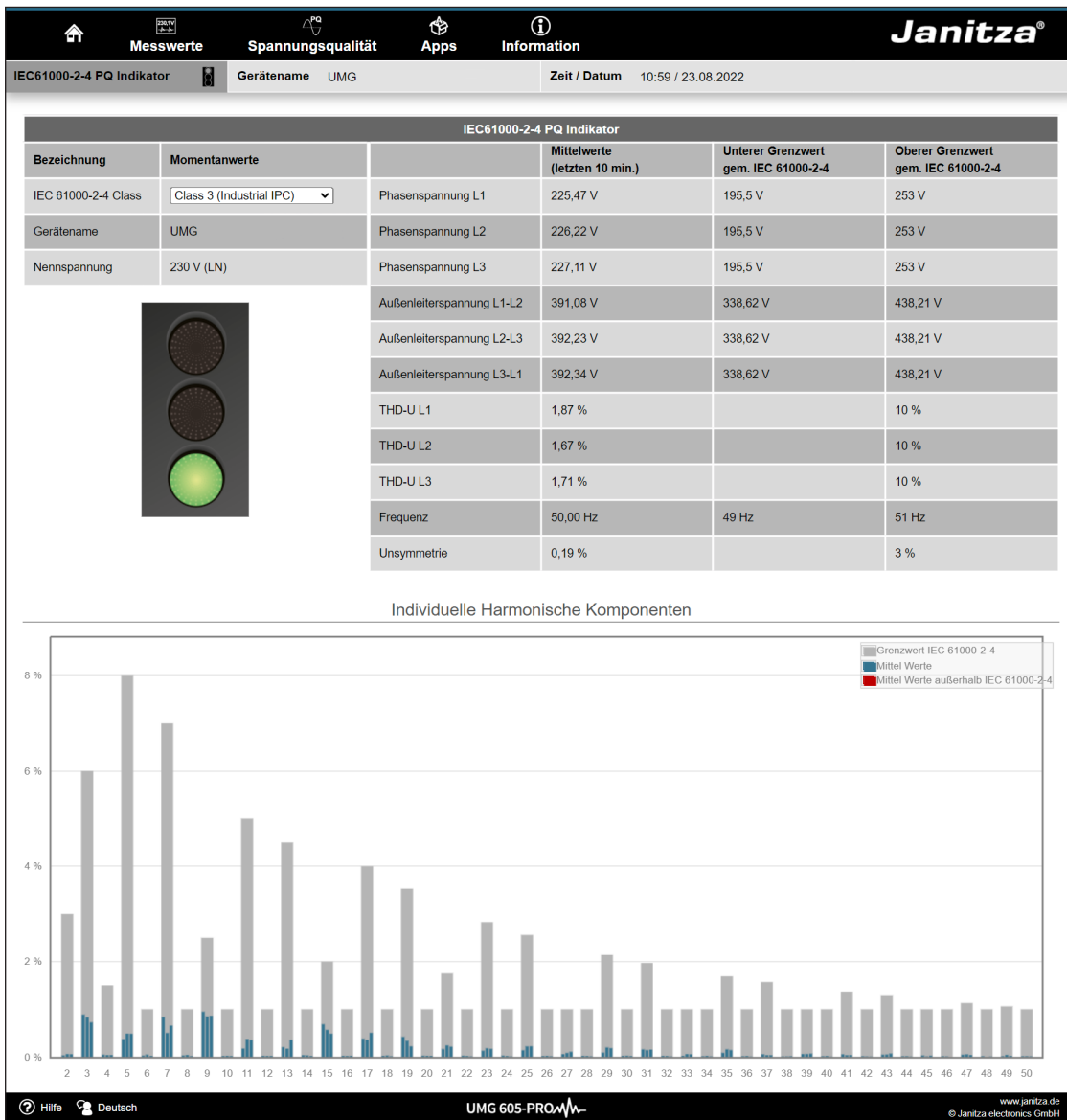
Abb. IEC61000-2-4 PQ Indikator Parameter mit Ampelprinzip - Momentaufnahme
