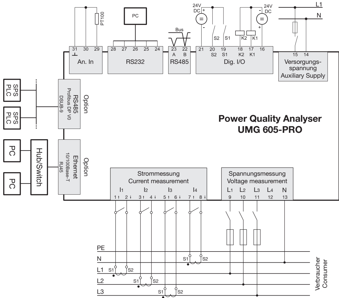
Abb. Anschlussbeispiel UMG 605-PRO
