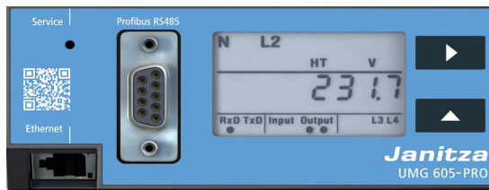
Abb. Frontansicht Bedienelement UMG 605-PRO
