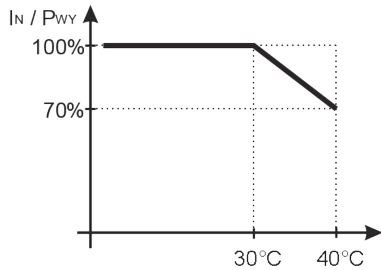
Schaubild 1: Zusammenhang zwischen Umgebungstemperatur und Ausgangsstrom
