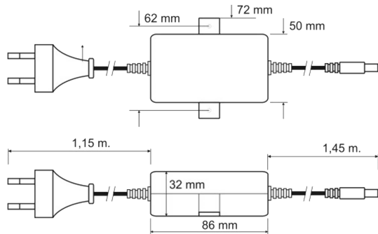
Abb. 1: Abmessungen
