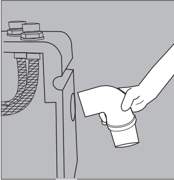
Anschlussbeispiel
