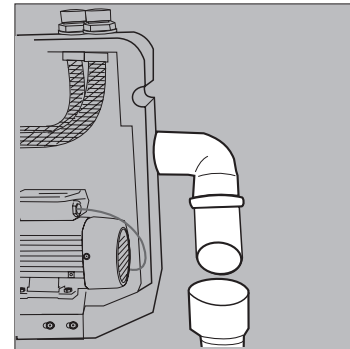
Anschlussbeispiel
