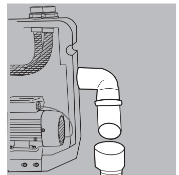
Entwässerungs- anschluss
