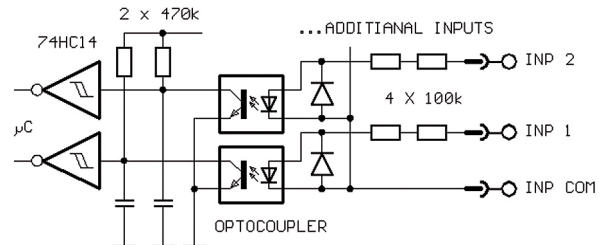
Abb. 3: Schaltbild Eingang
