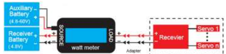
Vermessen der Empfangsanlage
