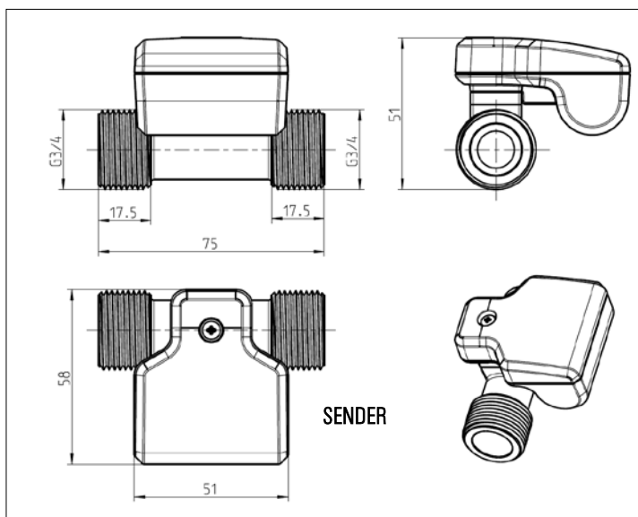
Funksystem, bestehend aus Sender und Empfänger (hier gezeigt Sender auf der Vision 3000)
