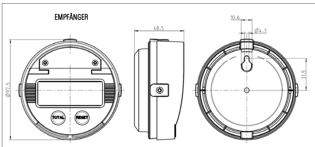
Funksystem, bestehend aus Sender und Empfänger (hier gezeigt der Empfänger)
