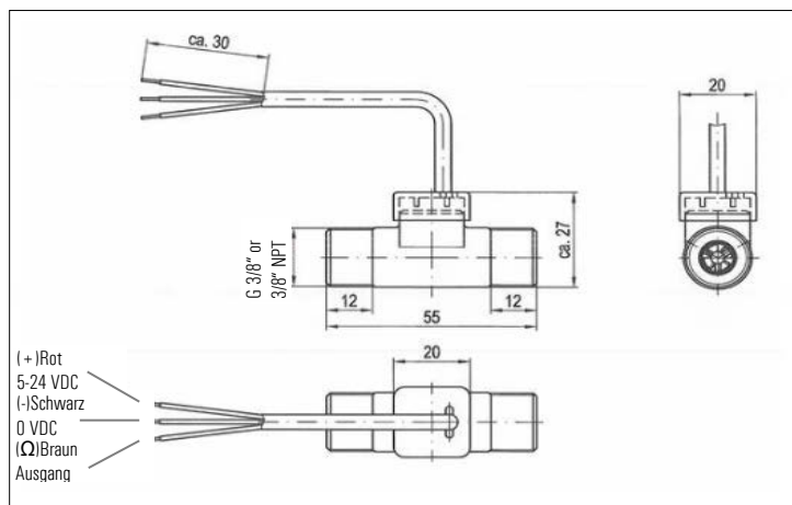
Beispiel: Vision 2000 mit Rundkabel 3 x AWG 24
