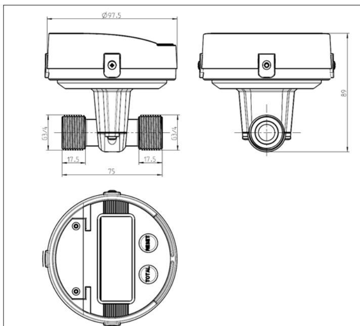
Beispiel Vision 3000 mit aufgebautem Display
