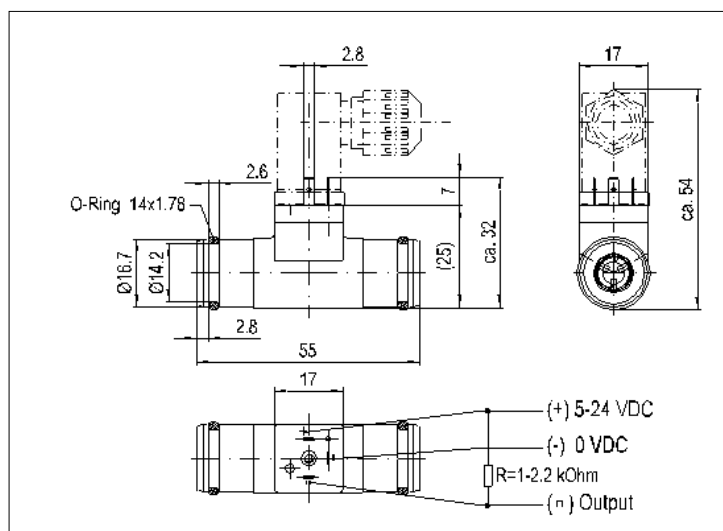
Beispiel: Vision 2000 mit O-Ring
