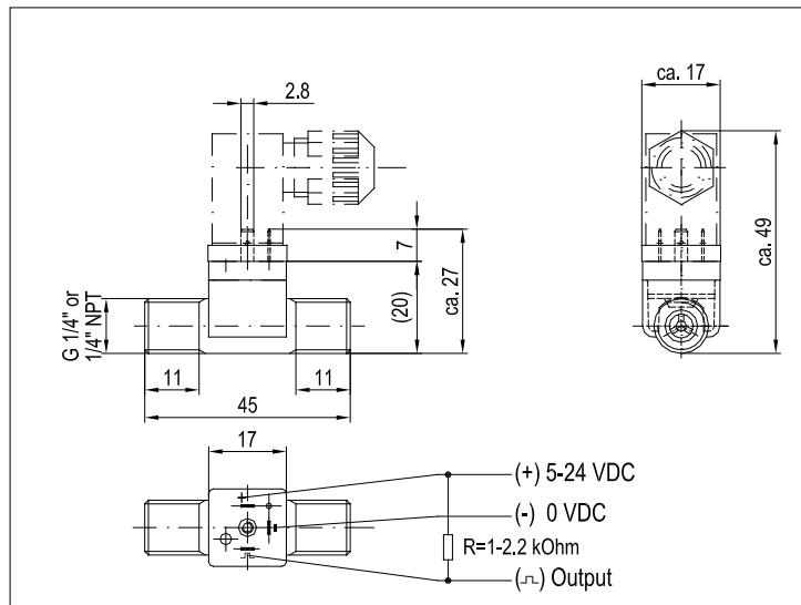
Beispiel: Vision 1000 mit DIN Stecker
