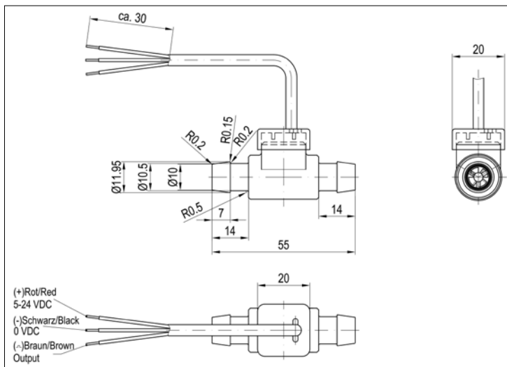
Beispiel: Vision 2000 mit Rundkabel 3 x AWG 24 und Schlauchnippel
