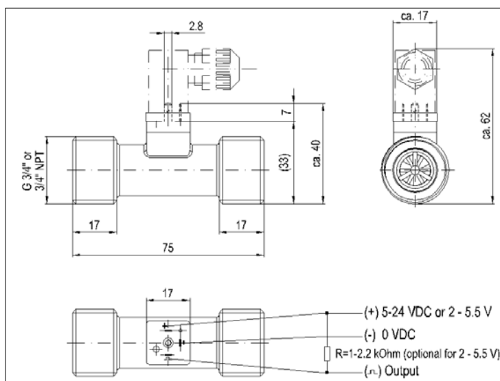
Beispiel: Vision 3000 mit DIN Stecker
