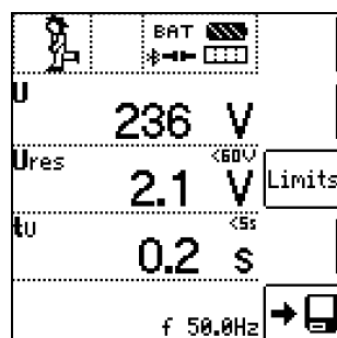
Anzeige Restspannungsmessung
