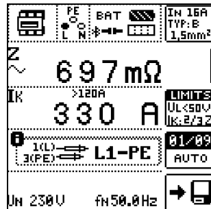
Anzeige Schleifenwiderstandsmessung
