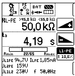
Anzeige IMD-Prüfung
