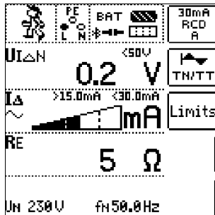
Anzeige RCD-Messung
