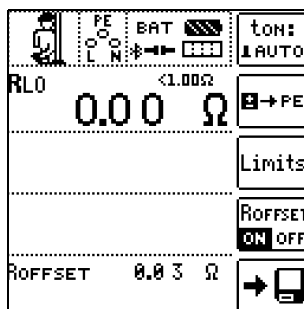
Anzeige Niederohmmessung 0,2 A
