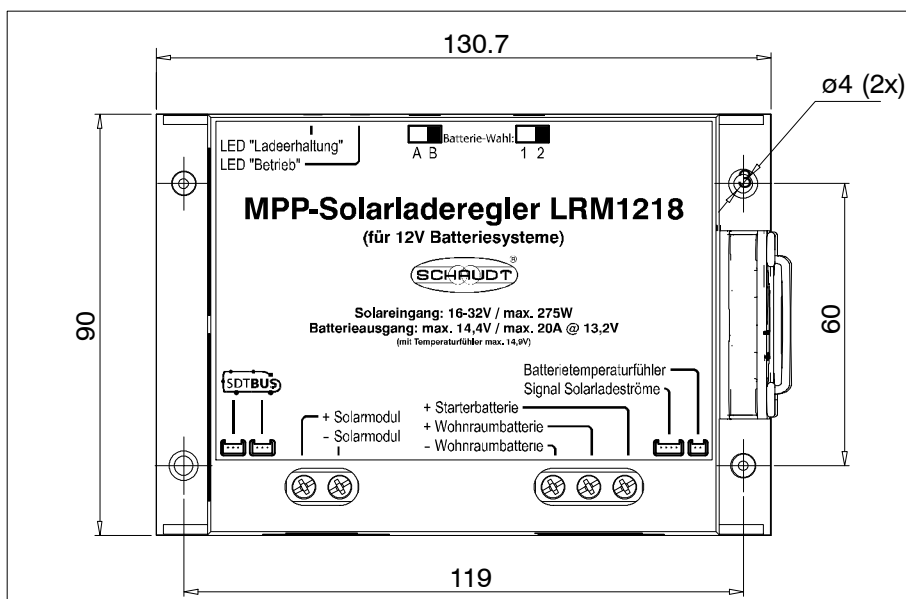
Bild 3 Befestigungspunkte Solar-Laderegler LRM 1218 (Abmessungen in mm)
