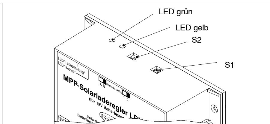
Bild 1 Schalter Batterieeinstellung und LEDs
