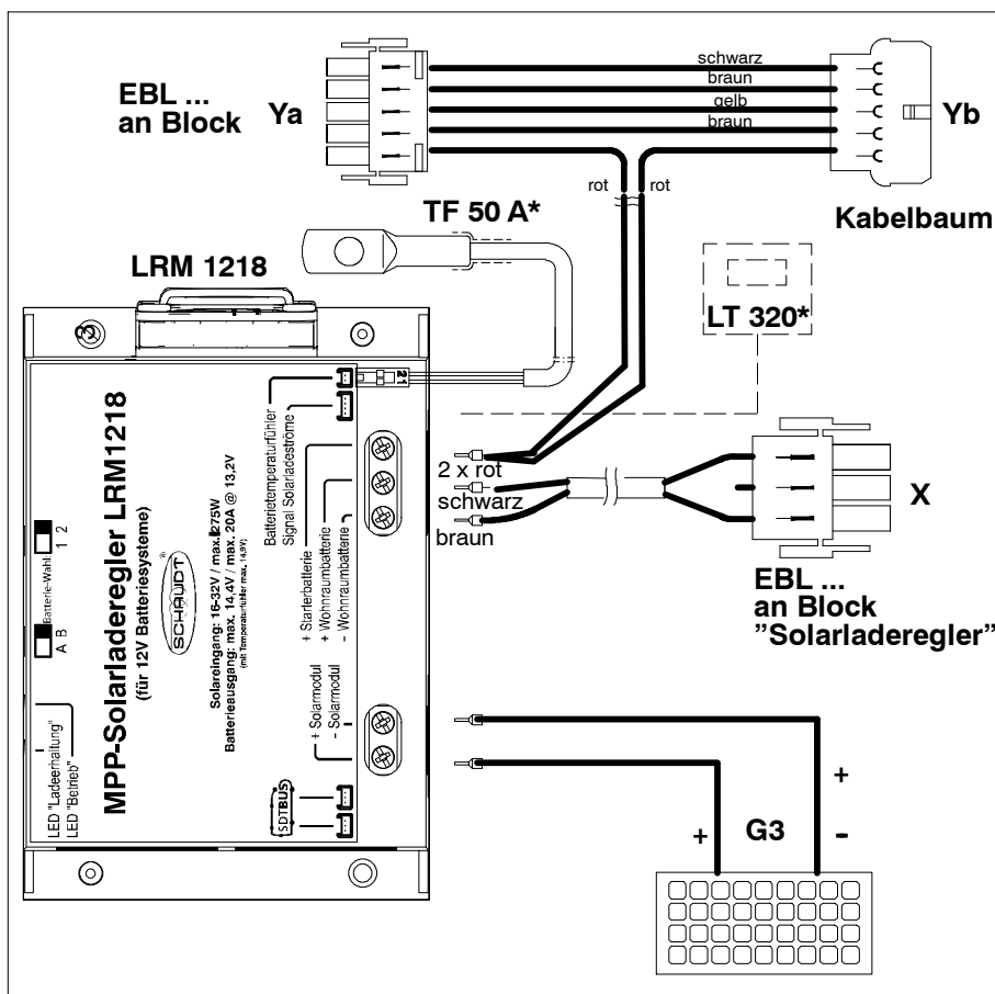
Bild 6 Schaltbild Anschluss LRM 1218 an EBL ...
