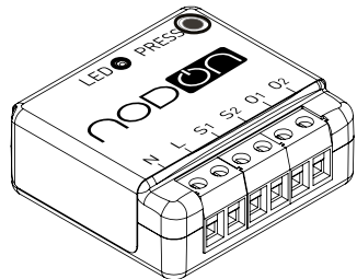
NodOn® Einbaumodul
