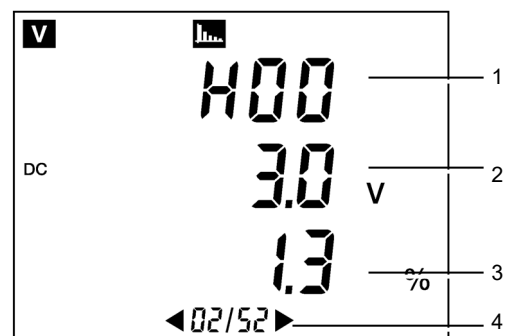
Abbildung 26: Beispielanzeige der Seite 2/52.
