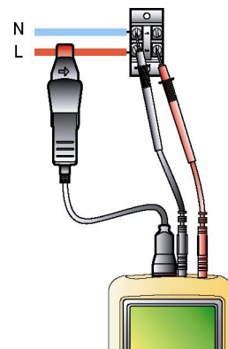
Abbildung 74: Einphasiger Anschluss. 005
