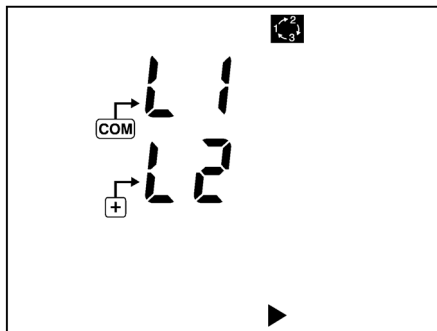
Abbildung 36: Der C.A. 8220 ist für die erste Messung zur Bestimmung der Phasenfolge betriebsbereit.
