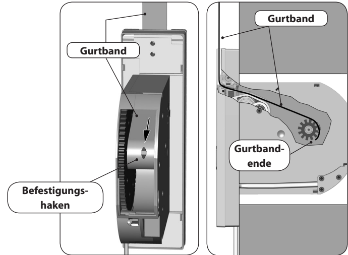
Gurtbandverlauf im RolloTron Standard DuoFern
