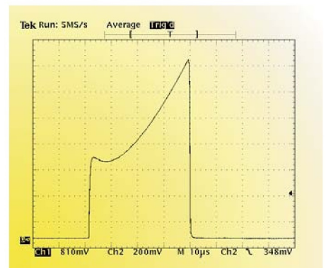
Ein 6700 A - Stromimpuls mit einem Abfall von 2700 A/µs, gemessen mit einer CWT 15 mit 500 mm Umfang und einem breitbandigen Koaxial-Shunt - 10 µs/div.
