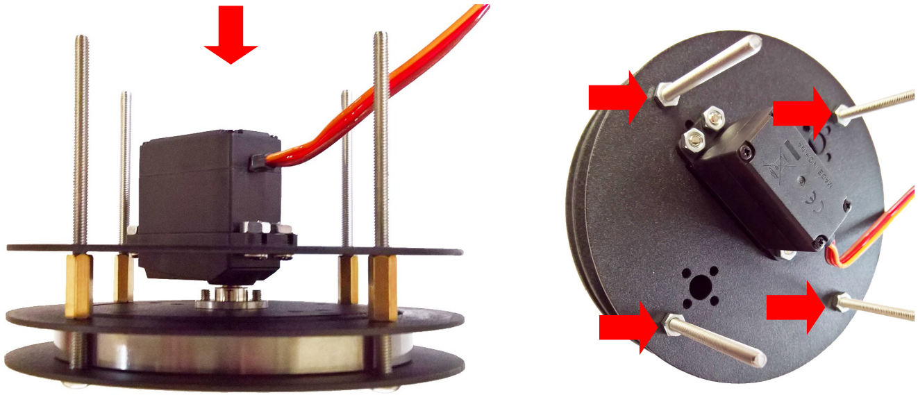
Die Platte mit dem Servo wird auf die Lagerhalterung aufgesetzt und mit 4 Muttern verschraubt.
