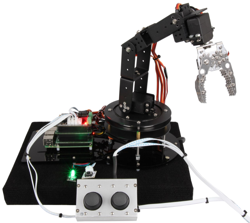
Abb. 1: Robot02 Inkl. optionalem Zubehör
