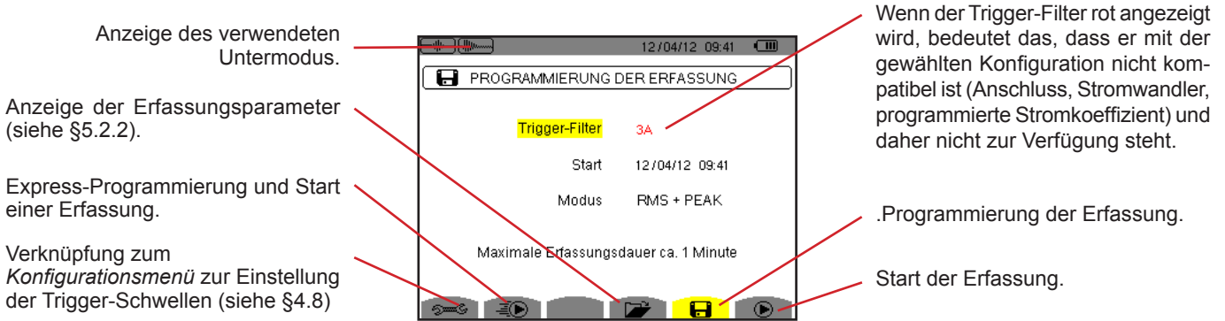
Abbildung 42: Bildschirm Programmierung der Erfassung im Modus Anlaufstrom
