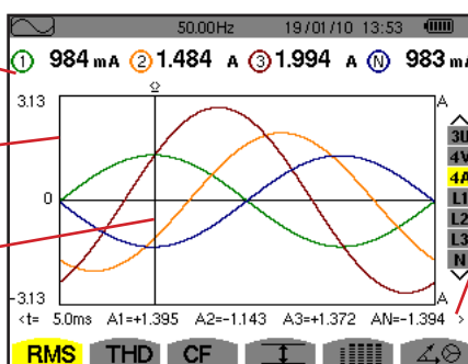
Abbildung 65: Bildschirm zur RMS-Anzeige bei 4A
