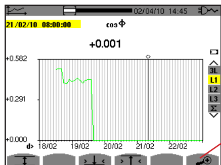
Abbildung 107: cos φ (L1) abgeschlossener Lade-/Berechnungsvorgang ohne MIN-AVG-MAX für eine dreiphasige Quelle mit Neutraleiter
