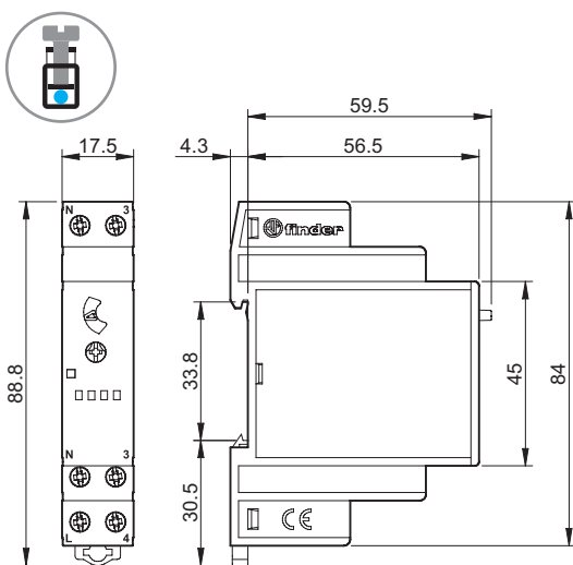
14.71 Schraubklemmen
