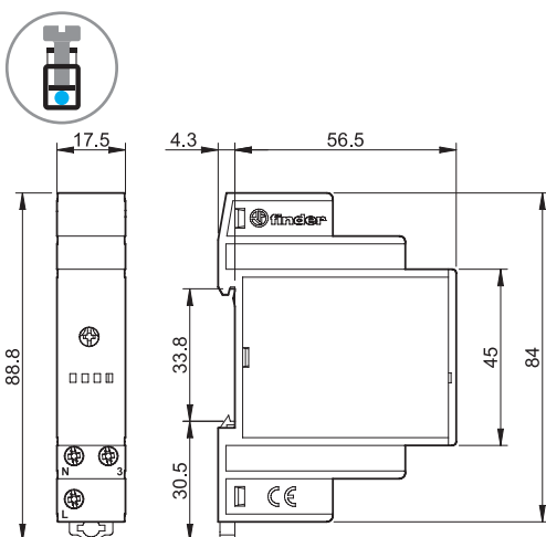
14.91 Schraubklemmen
