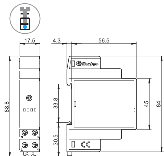
14.81 Schraubklemmen
