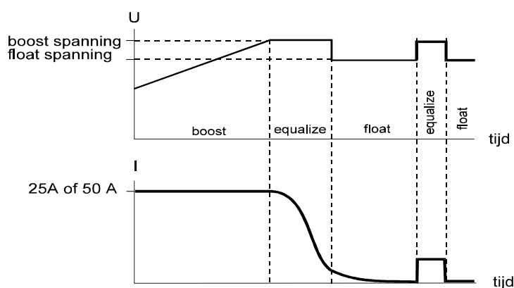
Abbildung 1. Die IUoUo-Lade- charakteristik
