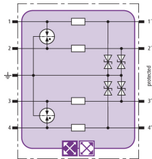
Prinzipschaltbild BXT ML4 BE 48
