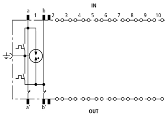
Principalschaltbild DRL 10 B FSD
