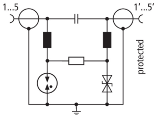
Prinzipialschaltbild DGA FF5 TV
