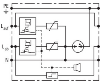
Prinzipschaltbild DCOR R 3P 275
