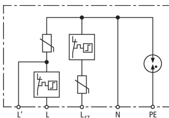
Principalschaltbild DCOR L 3P 275 SO IP
