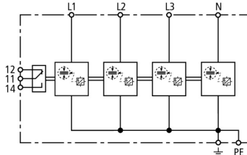
Prinzipschaltbild DSH TNS 255 FM
