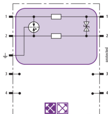
Prinzipschaltbild BXT ML2 BD 180
