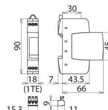
Maßbild DR M 2P 30 FM
