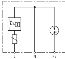
Prinzip Schaltbild DCOR L 2P 275
