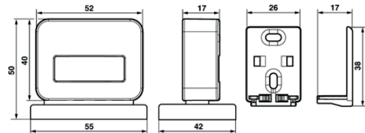
Abbildung 1: Abmessung in mm
