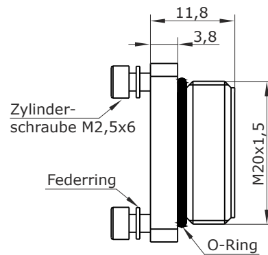
Hauptabmessungen Adapter
