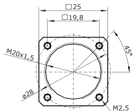
Hauptabmessungen Flansch
