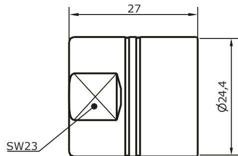
Hauptabmessungen Klemmringadapter
