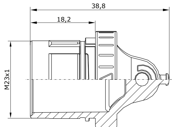
Hauptabmessungen Verschlussstopfen
