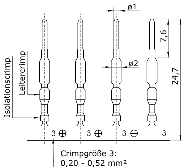
Hauptabmessungen Kontaktstift
