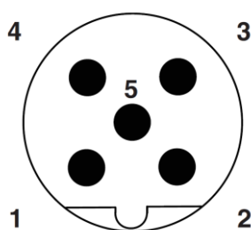
M12-Stecker, 5-polig, B-kodiert
