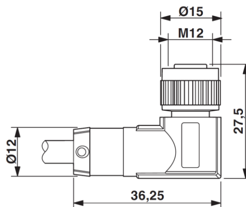
Maßzeichnung
