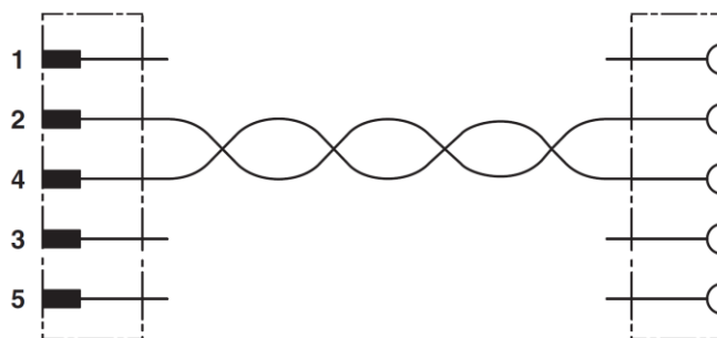
Kontaktbelegung des M12-Steckers und der M12-Buchse
