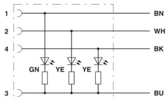
Schaltplan
