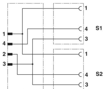
Schaltplan
