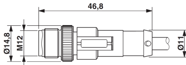
Stecker M12x1, gerade, geschirmt
