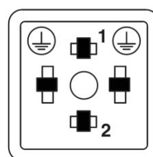
Polbild Ventilstecker, Bauform C
