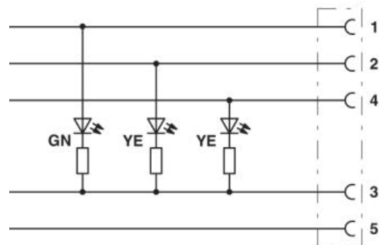
Schaltplan
