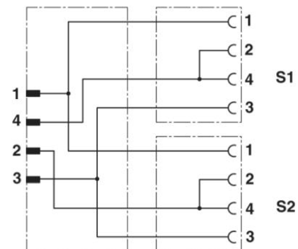
Schaltplan
