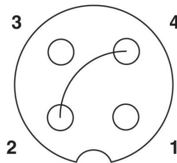
Schaltplan
