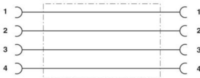
Schaltplan Kontaktbelegung der M12-Buchsen
