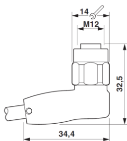
Buchse M12 x 1, gewinkelt
