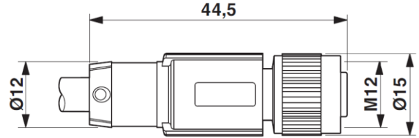
Buchse M12x1, gerade, geschirmt
