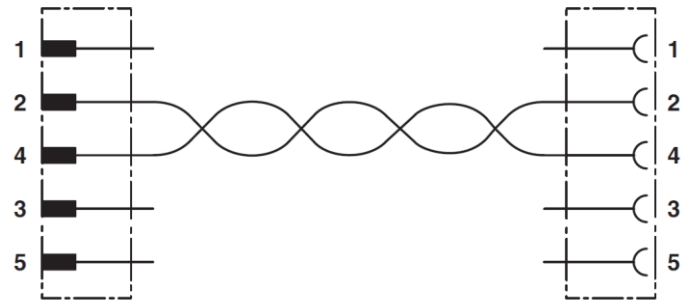
Kontaktbelegung des M12-Steckers und der M12-Buchse
