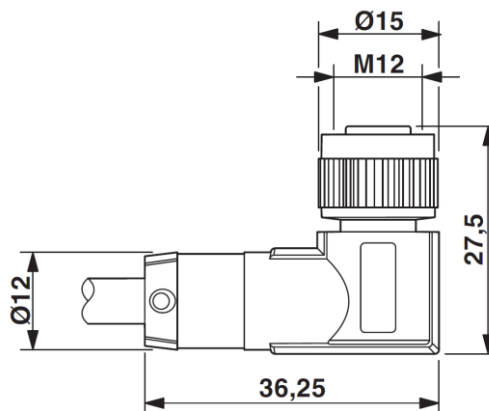
Maßzeichnung
