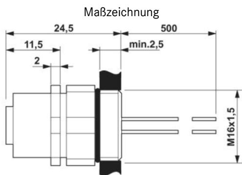
M12-Einbaustecker, positionierbar
