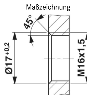
Gehäuseausschnitt für M16-Befestigungsgewinde, Montagewand mit Gewinde
