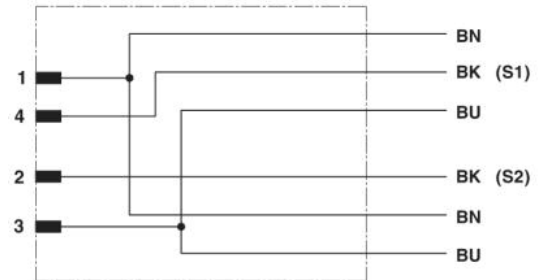
Schaltplan
