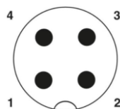
Polbild M12-Stecker, 4-polig, A-kodiert
