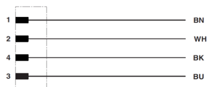
Kontaktbelegung des M12-Steckers und der M12-Buchse
